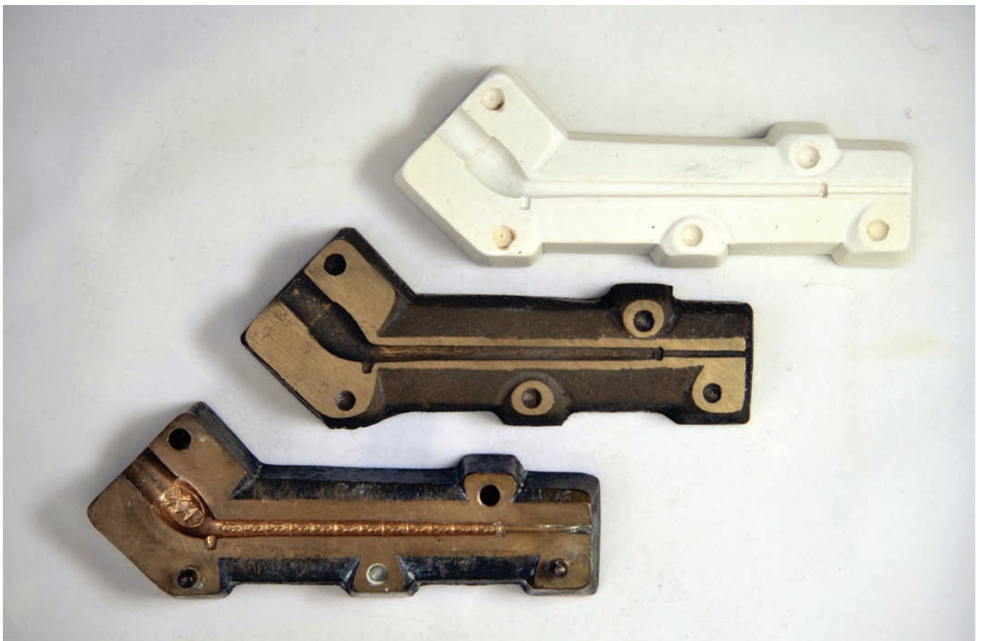
Afb. 19a-b. De ontwikkeling van de pijpjes die achtereenvolgens voor Verwoerd gemaakt zijn en de daarvoor door Cornelis Verwoerd gemaakte mallen. Het onderste pijpje is vermoedelijk gegoten. Collectie en foto Leo Verwoerd.
